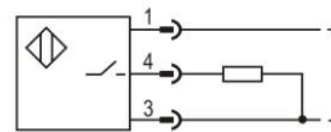
PNP NO
